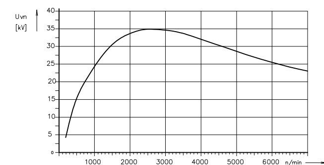
CHARAKTERISTIKA VYSOKÉHO NAPĚTÍ Zátěž 1M Ω / 50pF
