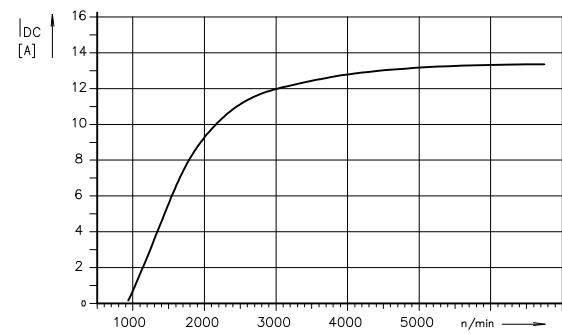
PROUDOVÁ CHARAKTERISTIKA SOUPRAVY U=14V-konst
